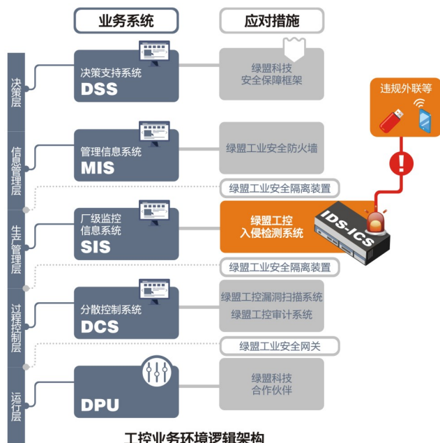
工控业务环境逻辑架构
